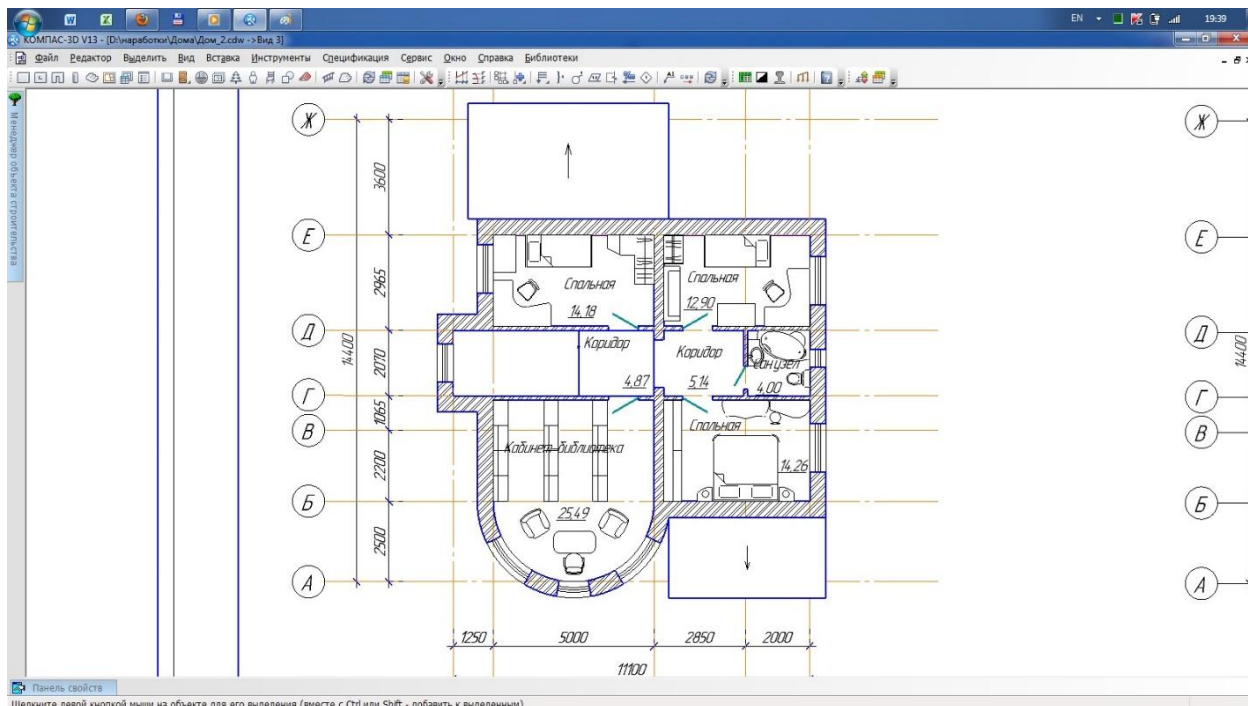
Рис. 2 план второго этажа
